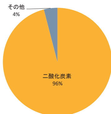
各温室効果ガスの構成比
